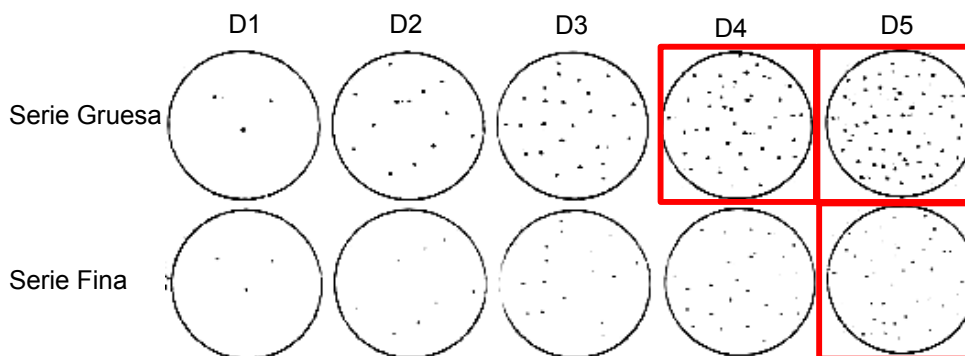
Figura B.2: Carta comparativa del nivel de inclusiones, según norma ASTM E45.
