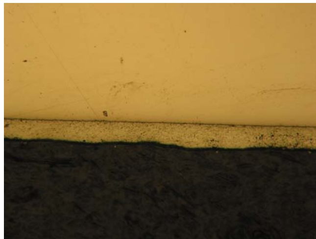
Figura B.3: 100X, sin ataque muestra T7/8, Espesor de la capa galvanizada.
