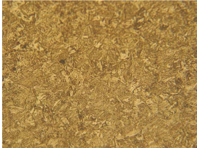
Figura B.4: Micrografía a 500 aumentos muestra T7/8.
